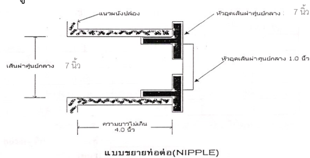
รูปที่ 5 แบบขยายของนิปเปิ้ล (Nipple) ของพอร์ตเก็บตัวอย่างแต่ละพอร์ต
